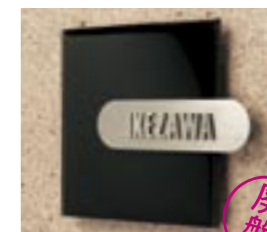
NS-SSG01 M6363 ￥— 235×200×23mm 本体:ステンレス t=3mm ガラス t=10mm 文字:ステンレス t=3mm 使用書体:ME-48
